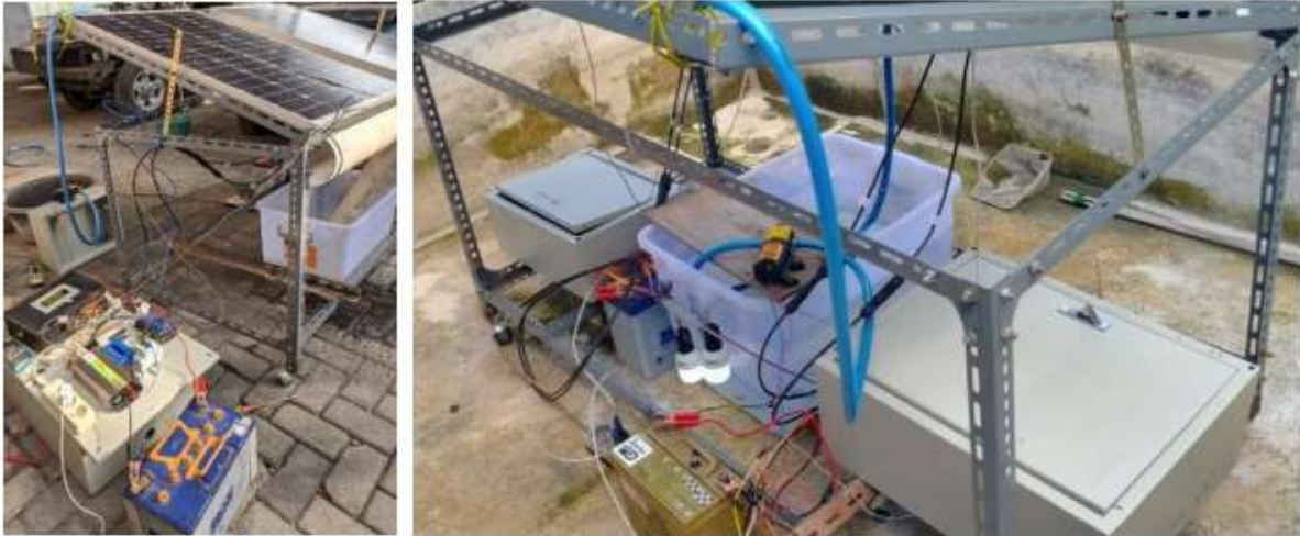
Gambar 2. Perangkat penelitian
