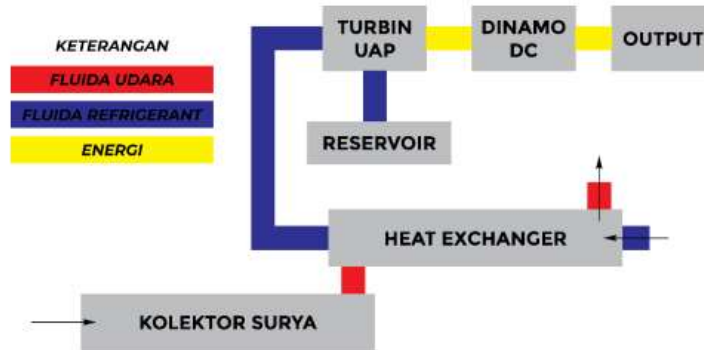
Gambar 2.1 Rancangan Prototipe PLTS Sitem Turbin Uap
