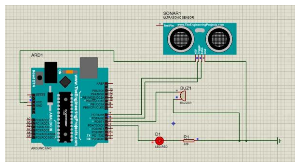
Gambar 6. Desain Sistem Sensor Parkir di Aplikasi Proteus 8 Professional
