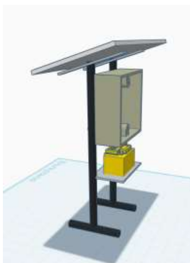
Gambar 2.5 Perancangan Server
