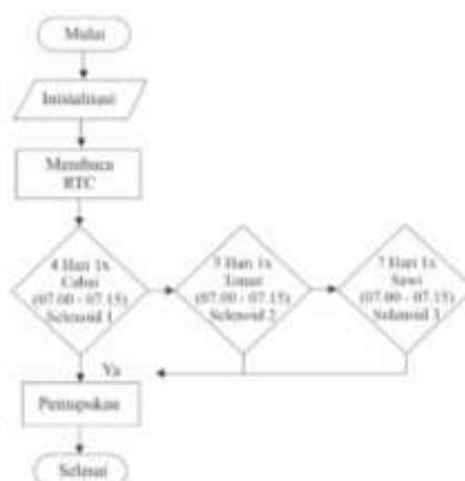
Gambar 4.3 Flowchart sistem pemupukan otomatis berdasarkan timer
